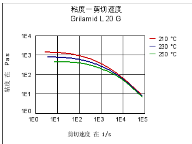
粘度 - 剪切速度
